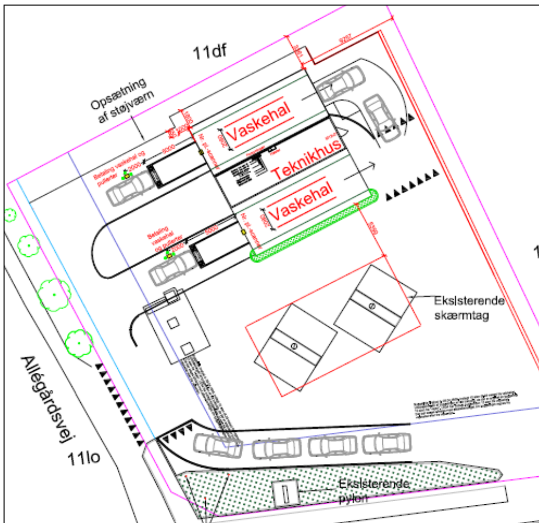
Situationsplan fra byggesag
