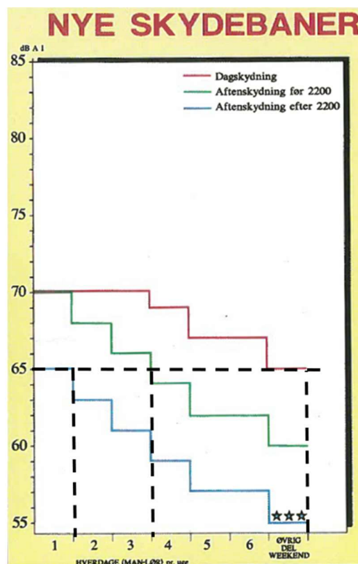
Figur 5: Retningslinjer for nye skydebaner. De stiplede linjer viser, hvad et støjniveau på 65 dB(A)I giver af skydetider.
