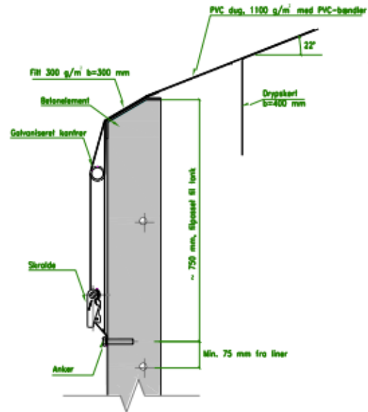
DETALJE A
