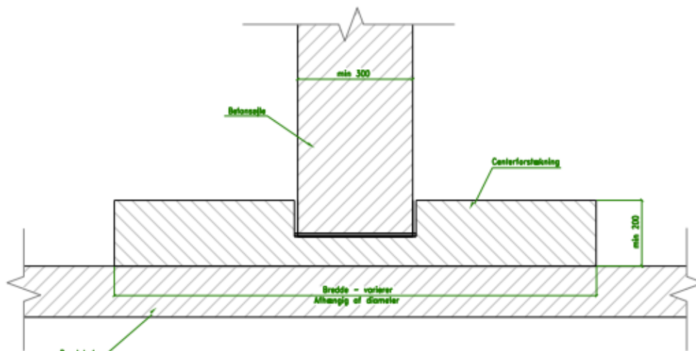
DETALJE B
