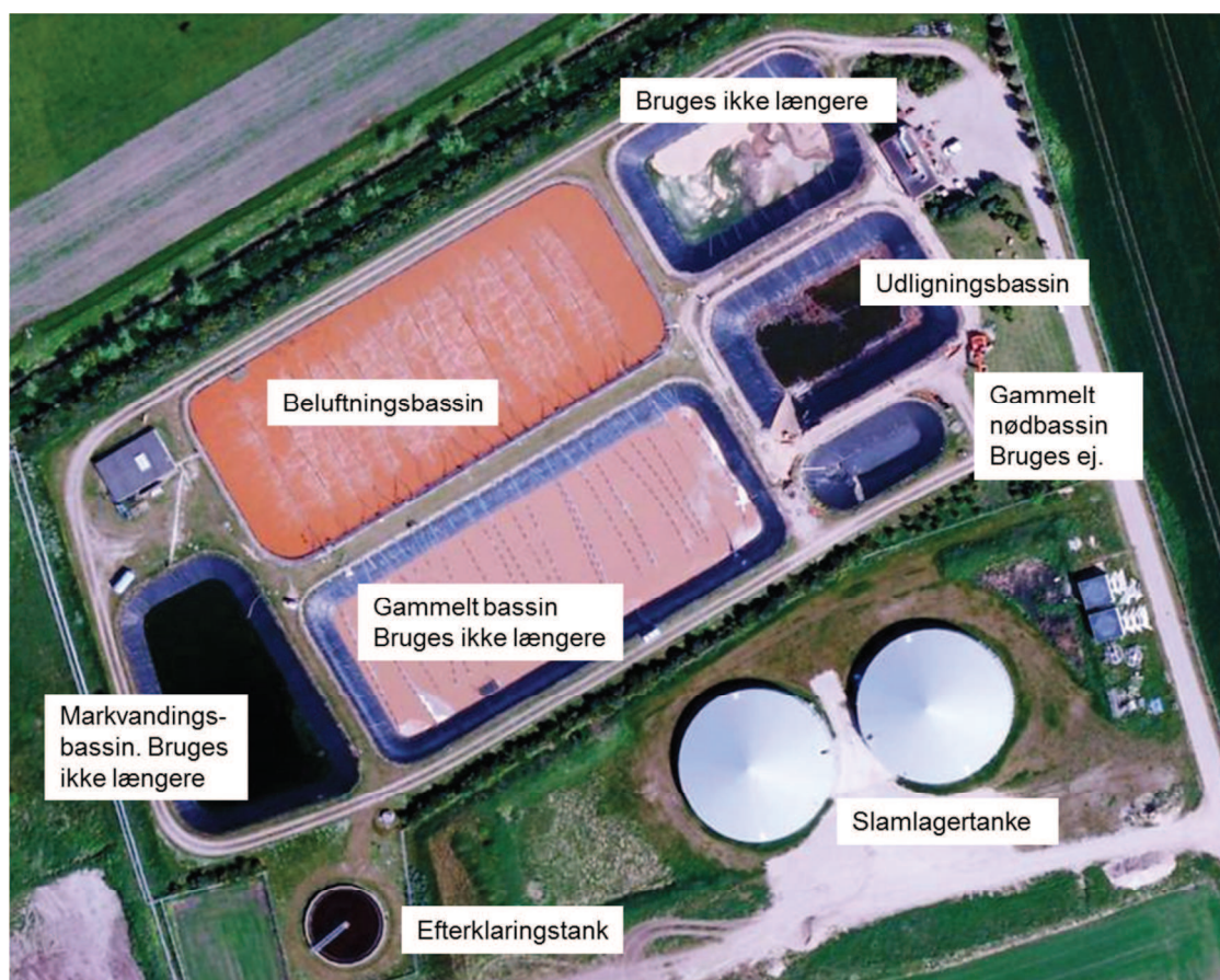
Figur 6.1 Spildevandsanlægget
