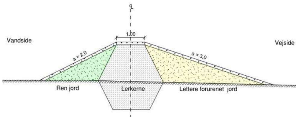
Figur 4: Udsnit af jordvoldens opbygning med impermeable lerkerne.
