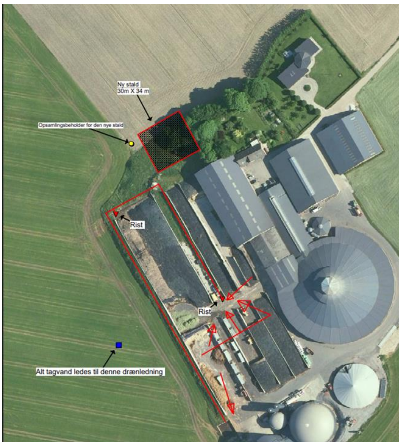
Figur 2. Spildevandsplan
