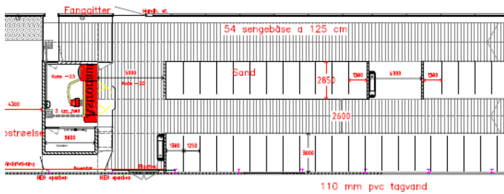
Malkerobotter og tilhørende teknikrum
