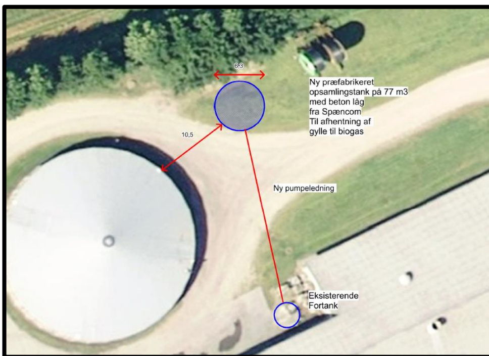
Figur 1. Placering af opsamlingsbeholder.
