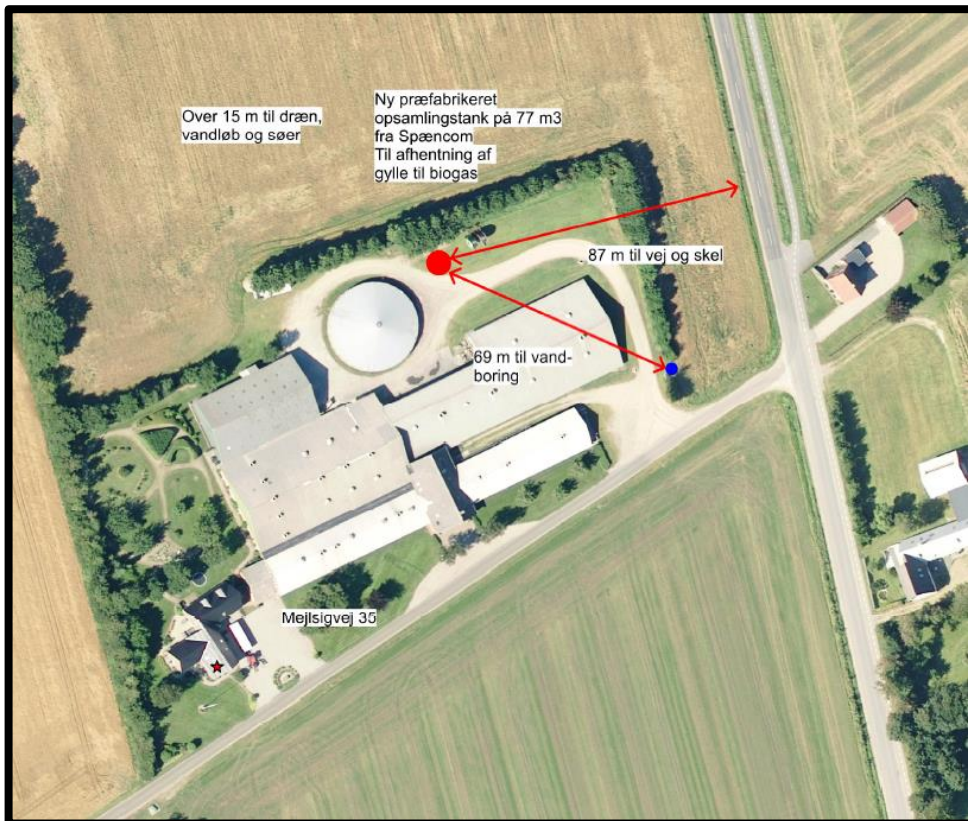
Figur 2. Placering af opsamlingsbeholder i forhold til skel og vandboring.
