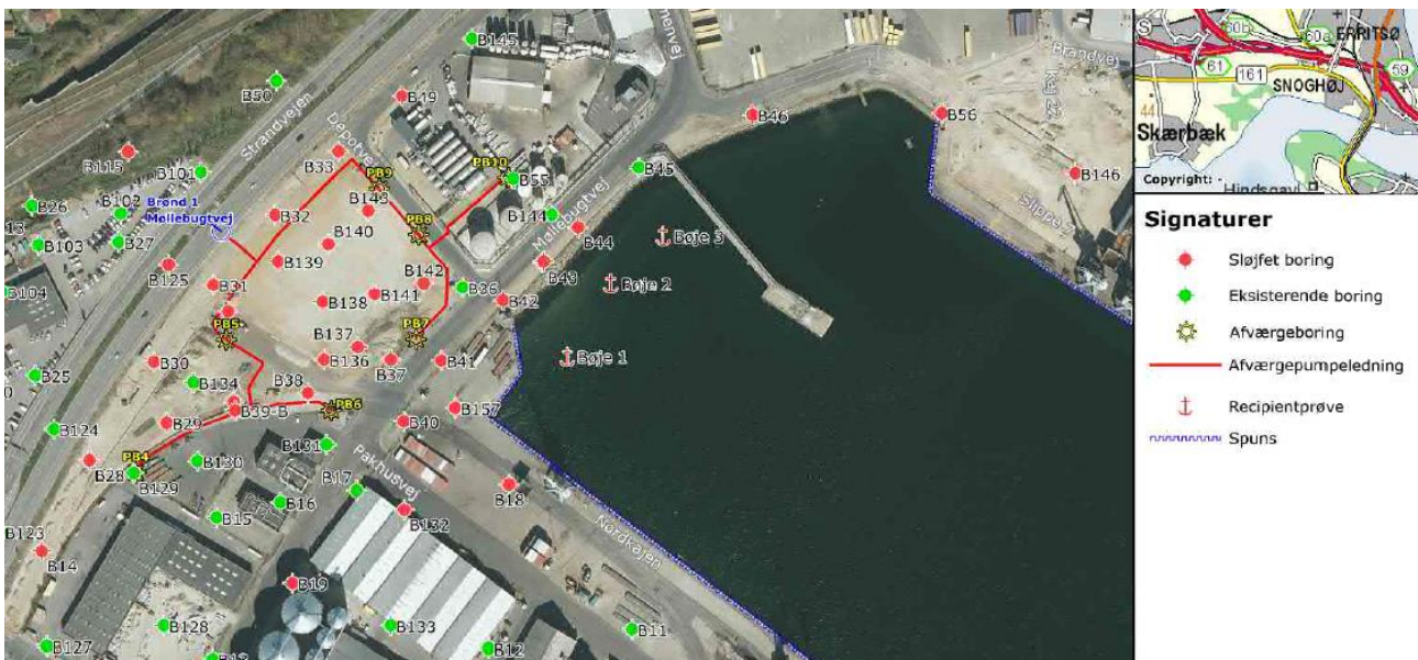
Figur 2: Placering af Dan Gødning afværgeboringer for fjernelse af kvælstof
