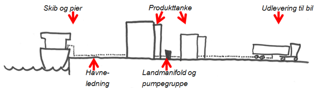
Figur 1 Skematisk illustration over terminalens opbygning
