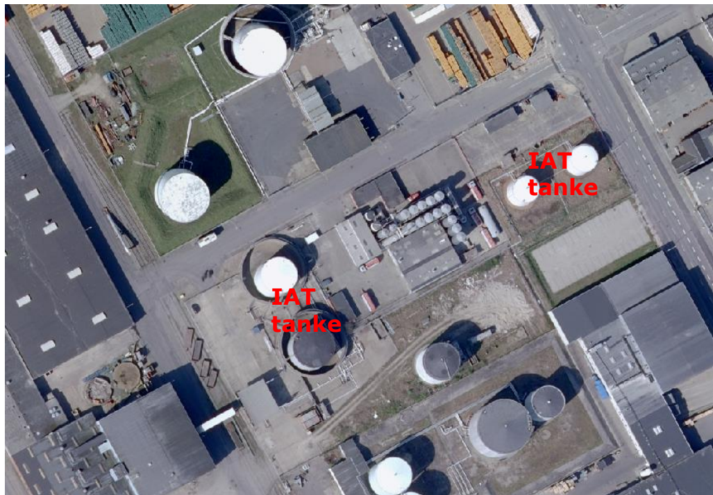
Figur 3 Overblik og placering af tanke i terminalen. Tankene er forbundet til en manifold med rørledninger, der er placeret over jorden.
