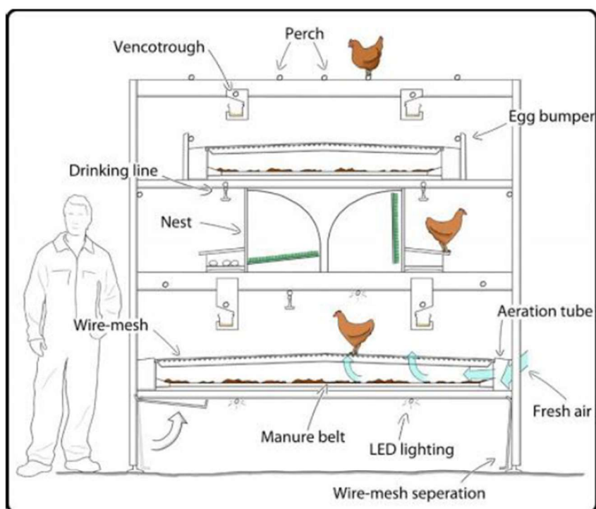
Figur 2. Teknisk tegning. Vencomatic Bole Terrace etageanlæg.
