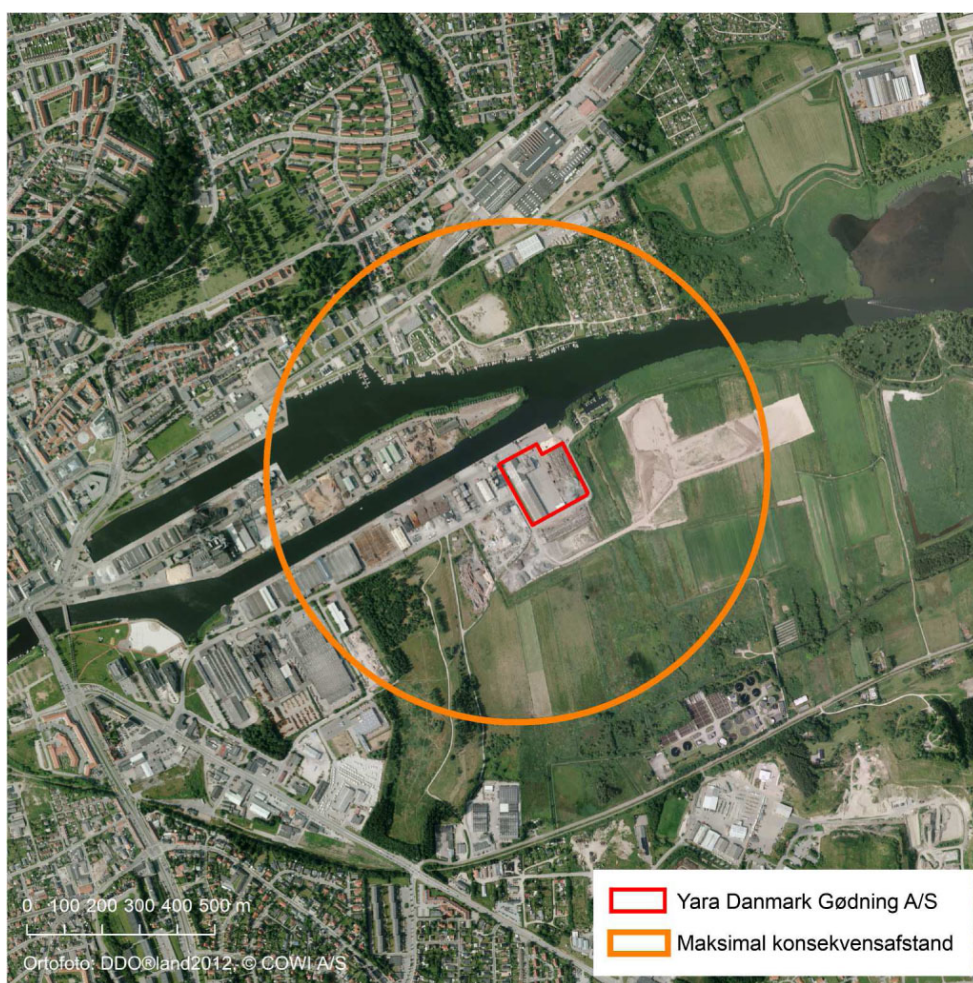
Figur 2: Maksimal konsekvensafstand
