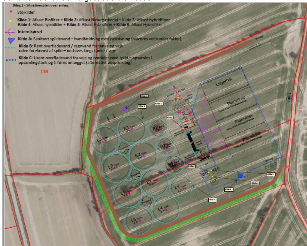
Figur 4; Situationsplan over anlægget
