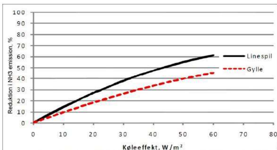
Figur 3. Forventet sammenhæng mellem køleeffekt, w/m² og ammoniakreduktion, % ved gyllekøling i svinestalde med hhv. skrabekanal og gyllesystem (Kai, 2009).
