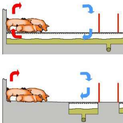
Figur 1. Skitser og sammenligning af ståndretning og typiske luftstrømme i stalde med henholdsvis drænet gulv og fast gulv i lejearealet.
