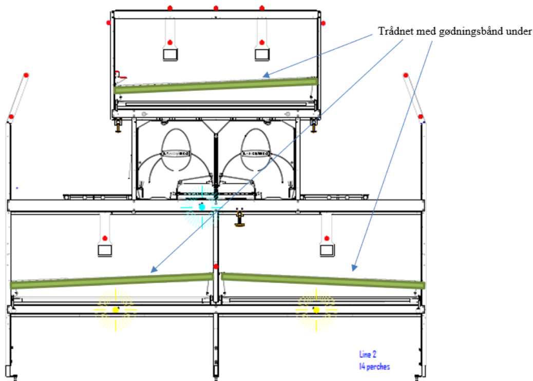
Figur 2 Produktionsarealer - markeret med grønt. Gulvet i hele stalden er også produktionsareal, når frihøjden under anlægget er min 45 cm.
