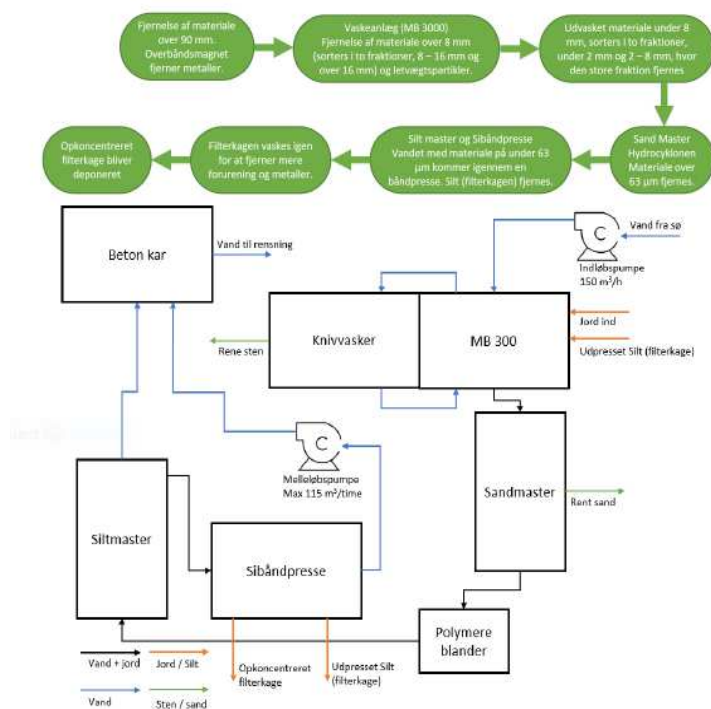
Figur 1: proces tegning af den fysiske kemiske og anlægget.
