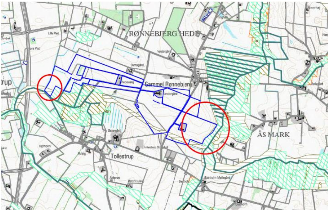
Figur N3. Udbringningsarealer (angivet med blå) der grænser op til beskyttede vandløb.
