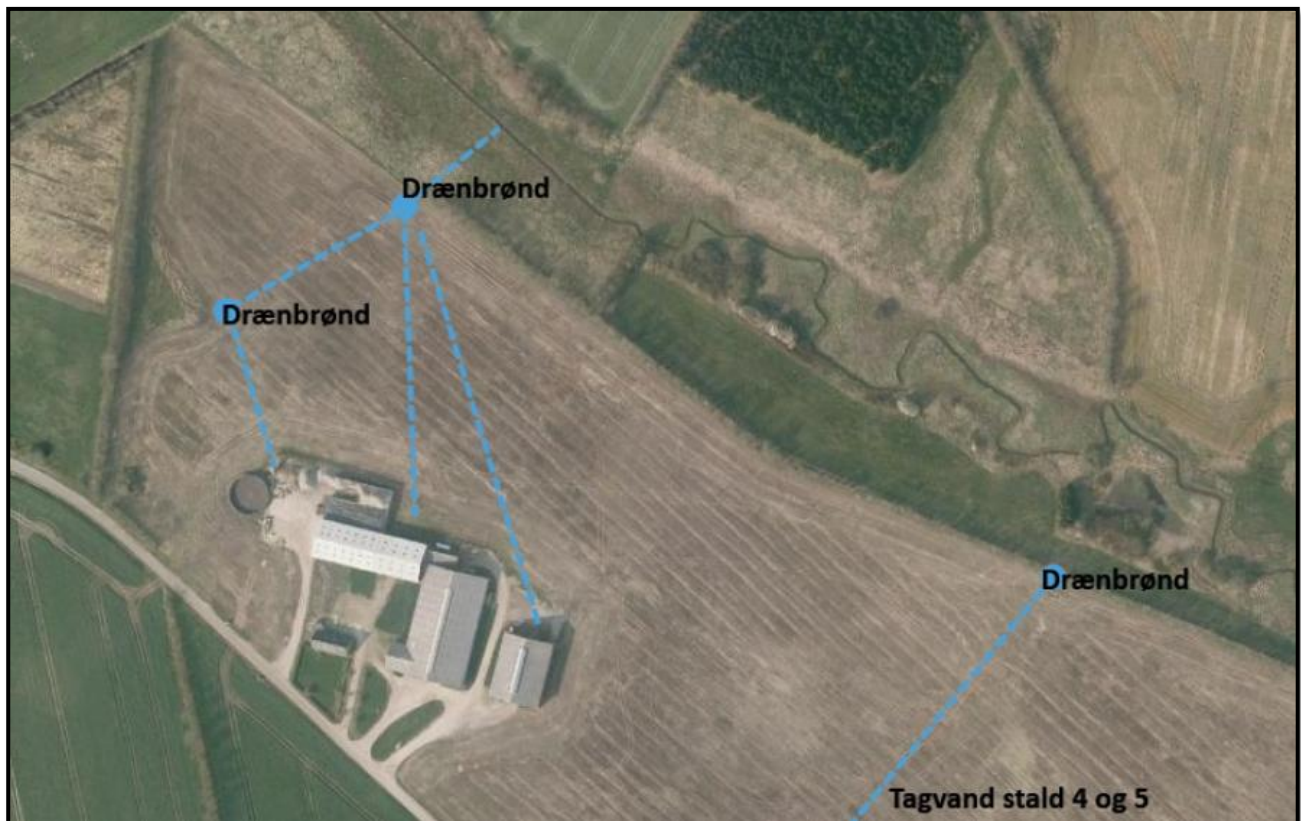
Figur 4. Afløbsplan og tagvand
