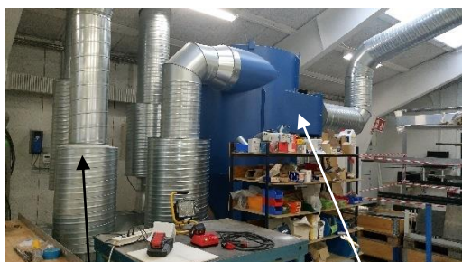
Billede nr. 1: Udsugningsanlæg for svejsning samt slibning og spåntagning (2020)
