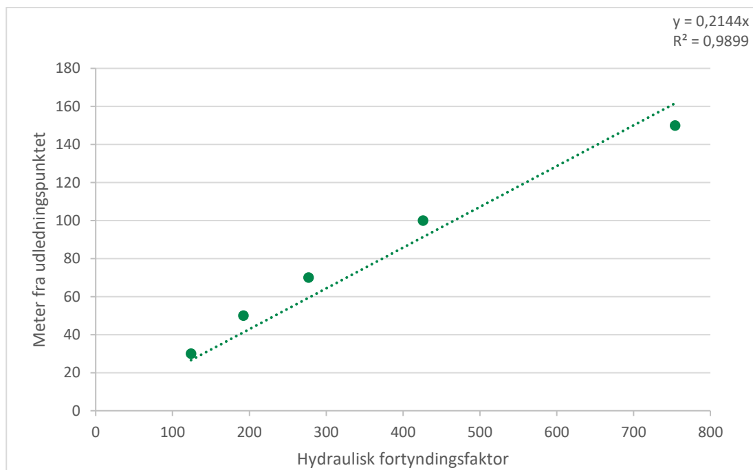
Figur 4.3 Lineær integration mellem afstand fra udledningspunktet for processpildevandet og beregnet hydraulisk fortynding.
