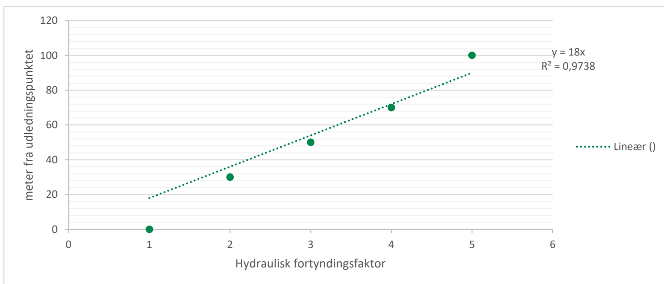
Figur 4.6 Lineær integration mellem afstand fra udledningspunktet for røggaskondensatet og beregnet hydraulisk fortyndingsfaktor.
