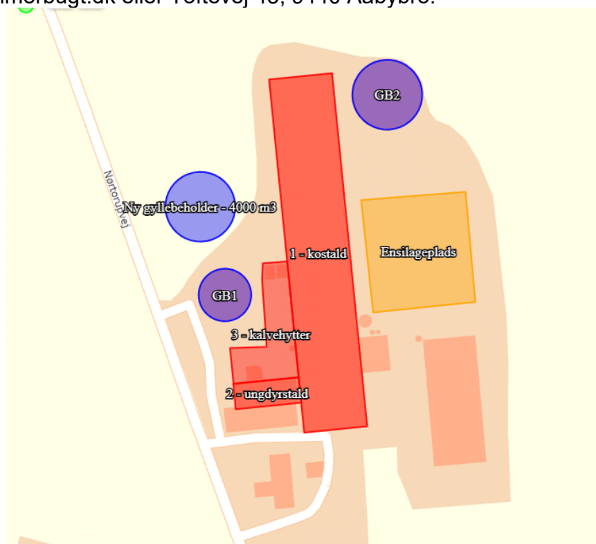
Figur 1: GB2 fjernes og erstattes af en den nye gyllebeholder
