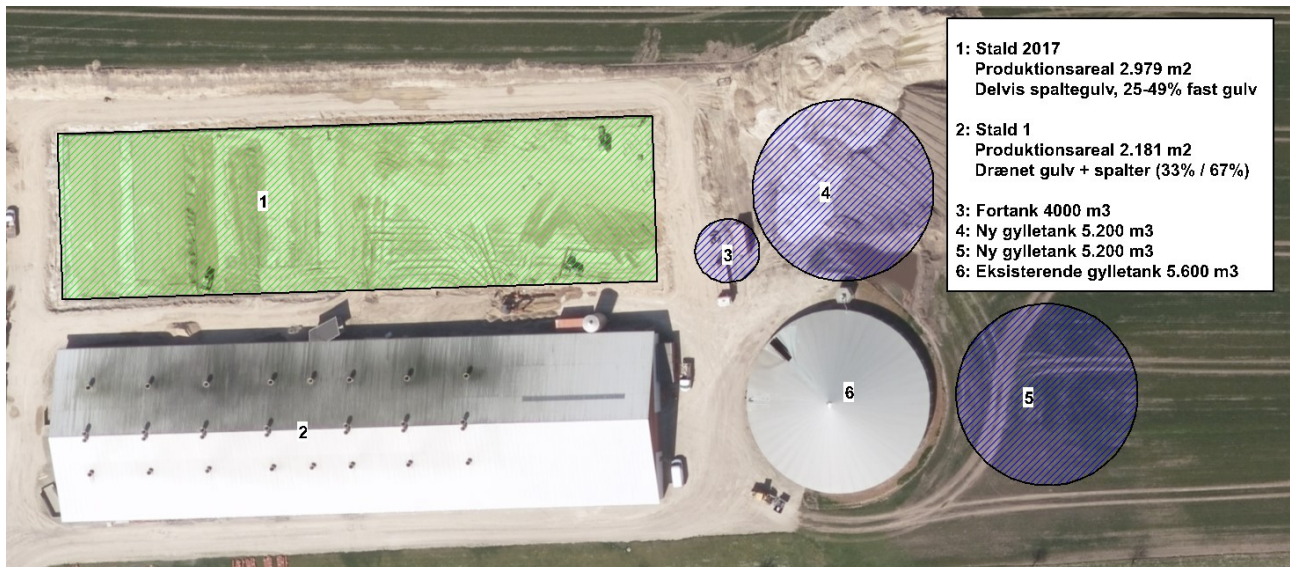
Billede 2 Bygningsoversigt med gulvtyper og produktionsareal
