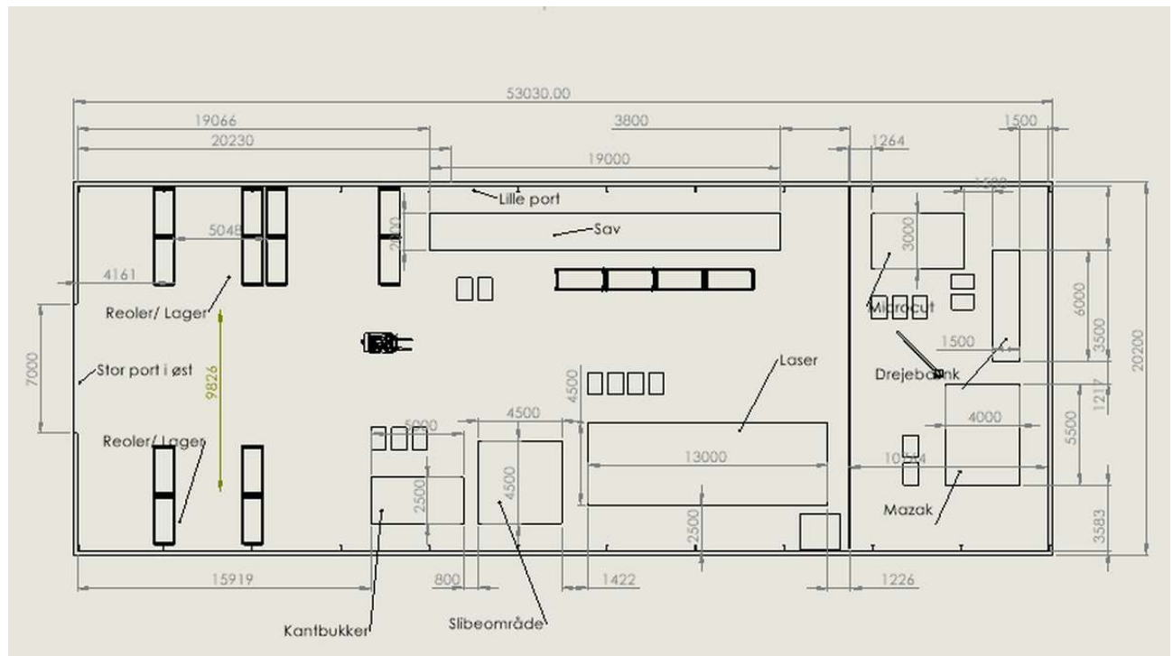
Situationsplan og indretning af maskinafdeling i del af hal M1
