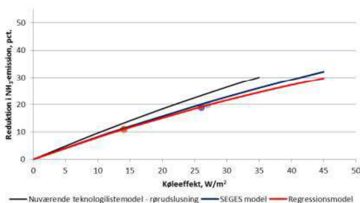
Figur 1. Sammenhæng mellem køleeffekt og ammoniakreduktion (% af ingen køling). Data stammer fra test af 10 slagtesvinestalde med rørudslusning, og hvor køleslangerne var nedstøbt i kummebunden.
