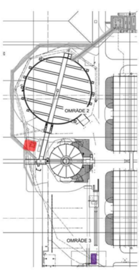
Figur 2 Skitse over de to siloer. Rødt område angiver udvidelse af eksisterende tankanlæg, lilla område angiver placering af brandvandspumpehuset (nederst i figuren).
