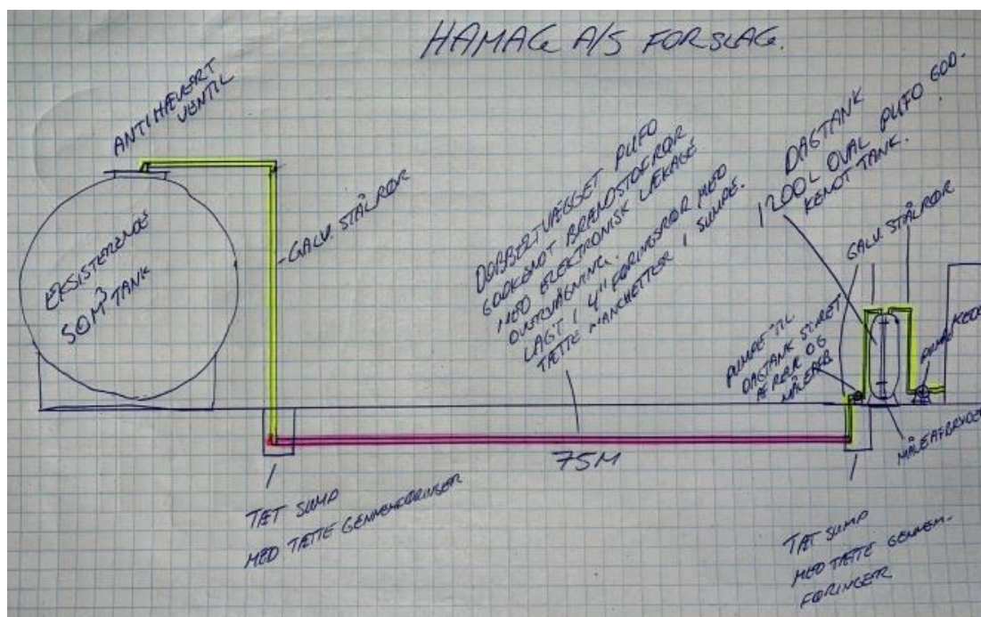
Figur 2: Billedet viser en skitsetegning over forbindelsen mellem den eksisterende brændstoftank og den nye dagtank.
