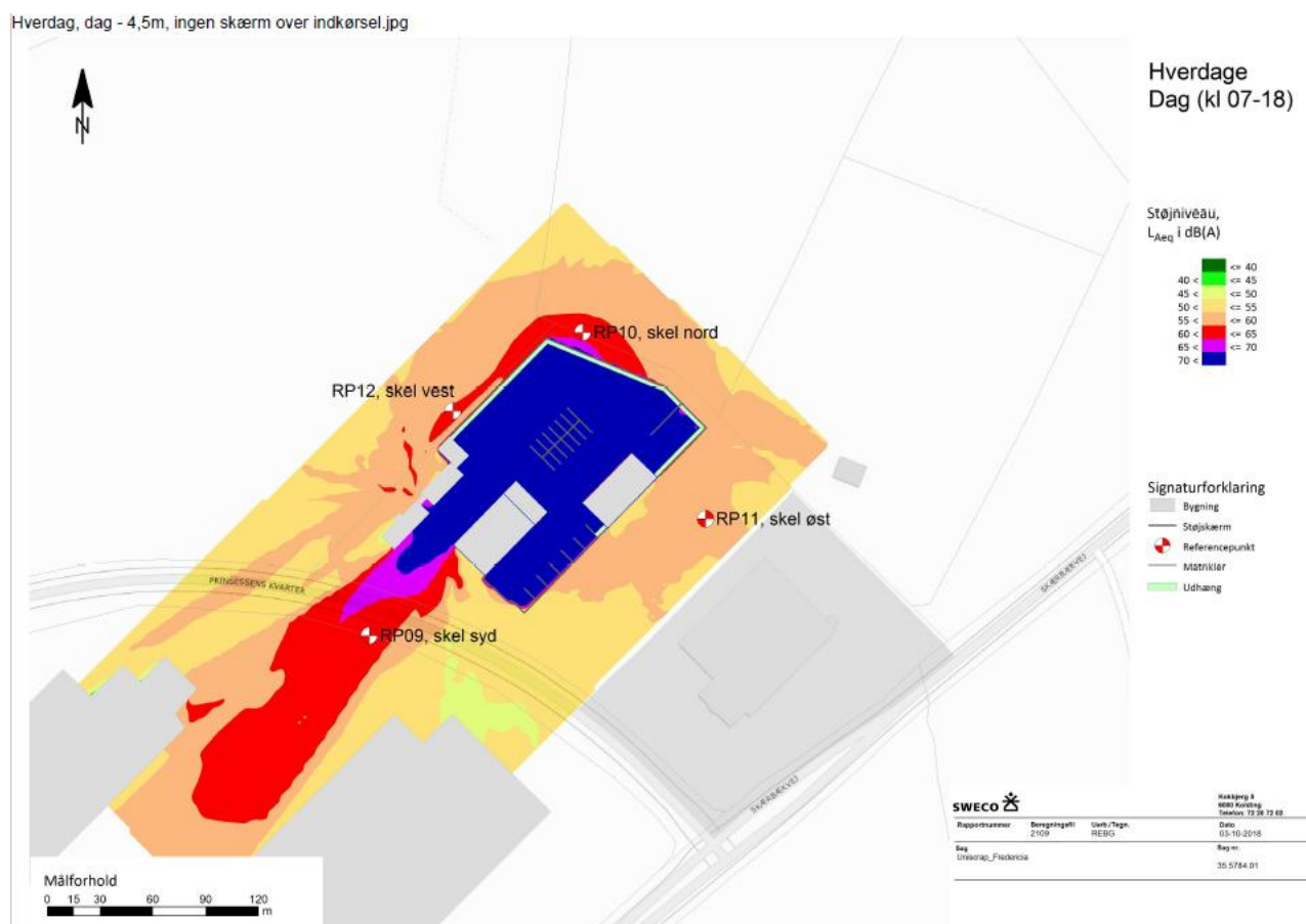
Figur 4. Støjudbredelseskort
