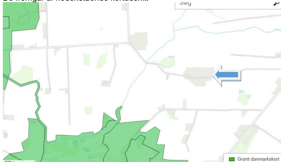
Figur 7. Blå 9il markerer placeringen af staldanlægget på Fåborgvej 15.
