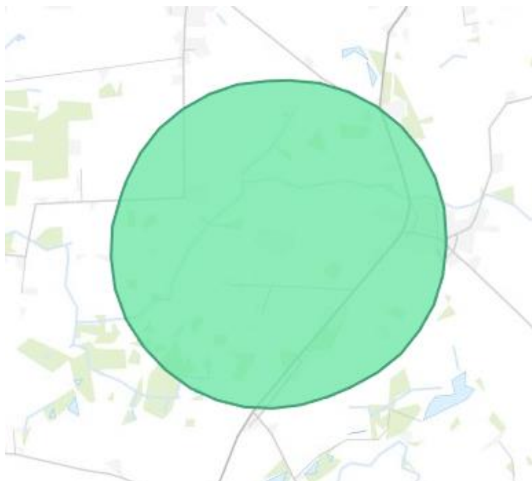
Figur A. Konsekvenszonen fremgår af markeringen på ovenstående figur.
