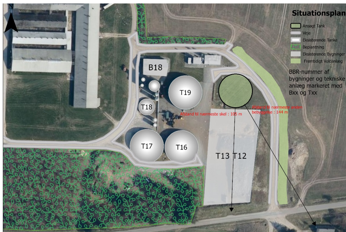
Figur 1 - Situationsplan med ny efterafgasningstank markeret med grønt
