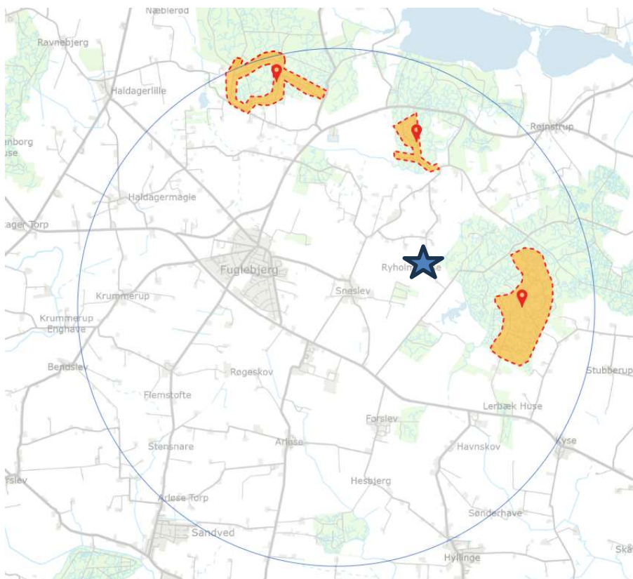
Figur I. De tre skovområder, hvor der er registreret flagermus (Danmarks Naturdata). Højbjergvej 10A er angivet med en stjerne.
