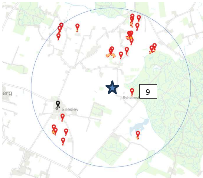
Figur j. Registreringer af stor vandsalamander og dens potentielle ynglevandhuller. Danmarks Naturdata. Ejendommen er markeret med stjerner.
