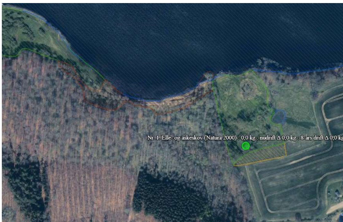
Figur c. Naturpunkt 1 med grøn prik. Gul skraveret er overdrev, hvor beregningspunktet burde have ligget.
