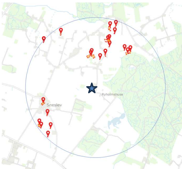
Figur i. Registreringer af springfrø og dens potentielle ynglevandhuller. Danmarks Naturdata. Ejendommen er markeret med stjerne.
