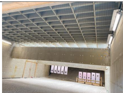
Foto 2 Støjbafler over pistolbane
