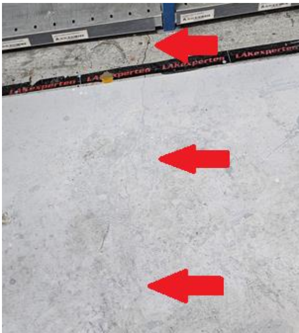
Revne i betongulv i rum med miljøfarlige stoffer.
