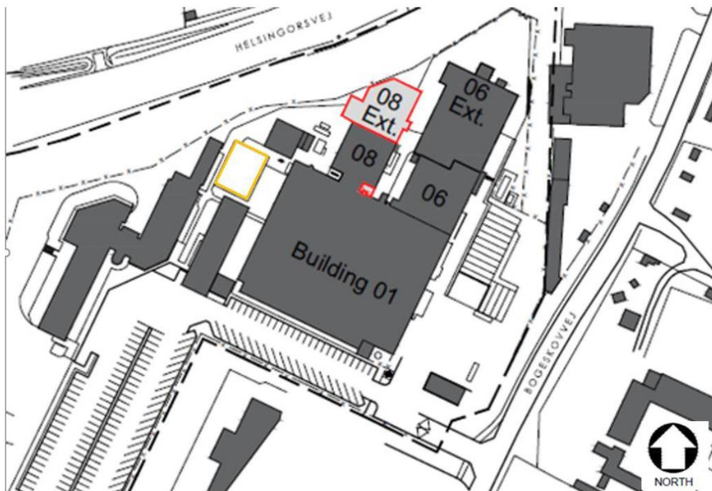
Figur 1 Princip plan. Tilbygningen til bygning 8 (08) er markeret med rødt, eksisterende kølegård er markeret med orange, hvor der vil blive etableret en ny utility-bygning for dampkedel og køleanlæg.
