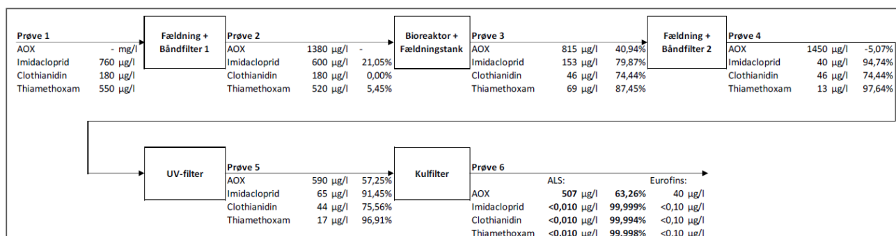
Figur 1: Diagram over renseeffektivitet for pesticider og AOX'er gennem Flux Waters renseanlæg opgjort i koncentration og akkumuleret rensegrad
