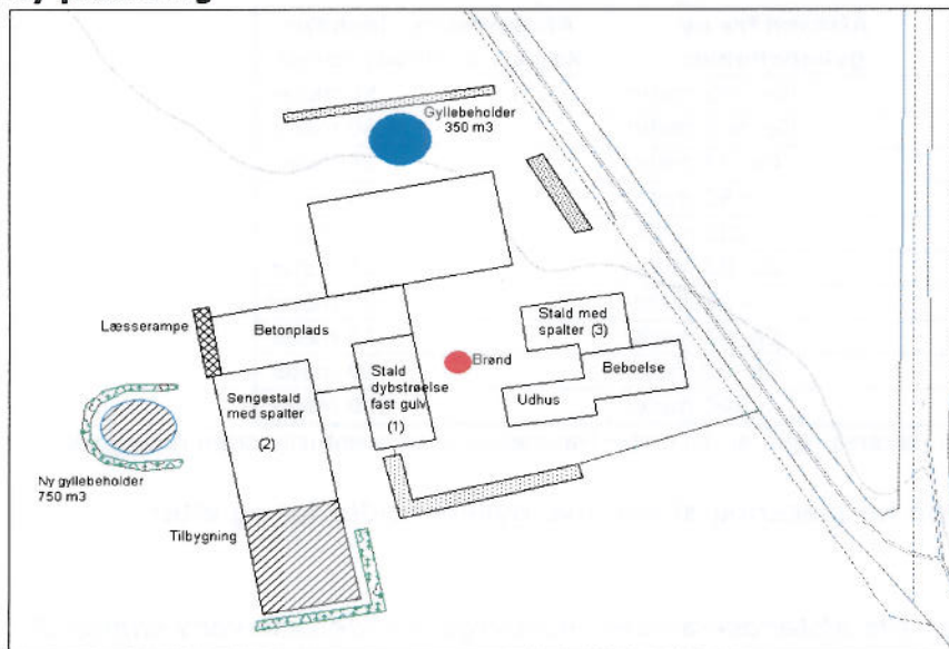
Figur 3: Oversigtstegning over husdyrbruget bygninger med angivelse af placeringen af den nye gyllebeholder. (ny afskærmende beplantning er det grøn skraverede område)
