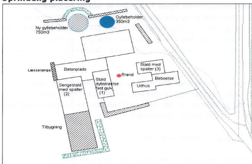
Figur 2: Oversigtstegning over husdyrbruget bygninger med angivelse af placeringen af den nye gyllebeholder i henhold til tidligere miljøtilladelsen.
