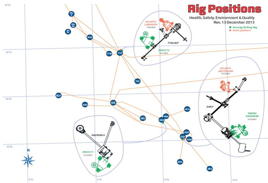
Figur 2 Illustration over rigges placering, her pr. december 2013. Grøn rig er borerig mens rød er beboelsesrig.
