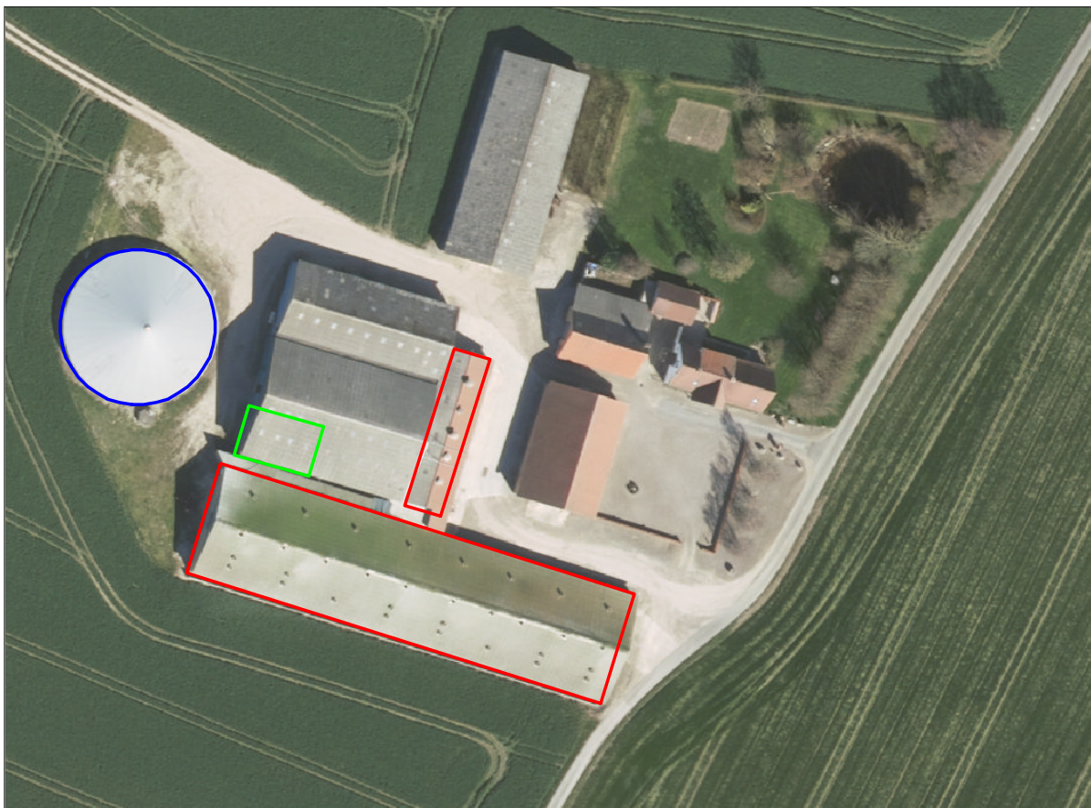
Indretning af husdyrbruget på Spanggårdsvej 2. Svinestalde er markeret med rødt og kvægstalde med grønt. Gylletanken er vist med blå.
