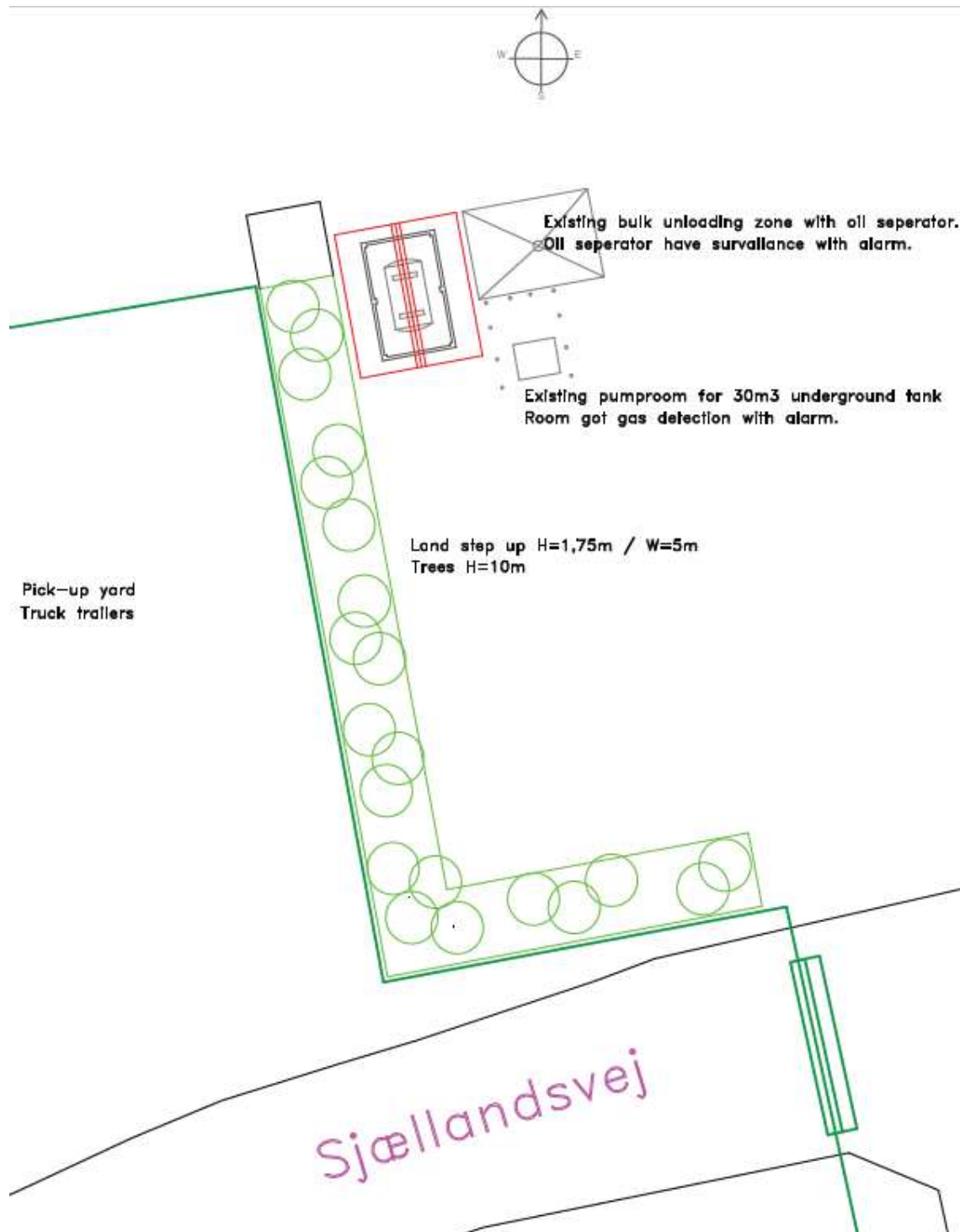
Figur 1 placering af ny tank til cyclopentan / isopentan.
