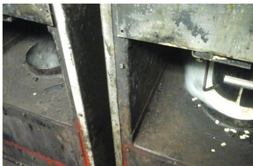
Røgkammeret, hvor smuld afbrændes
