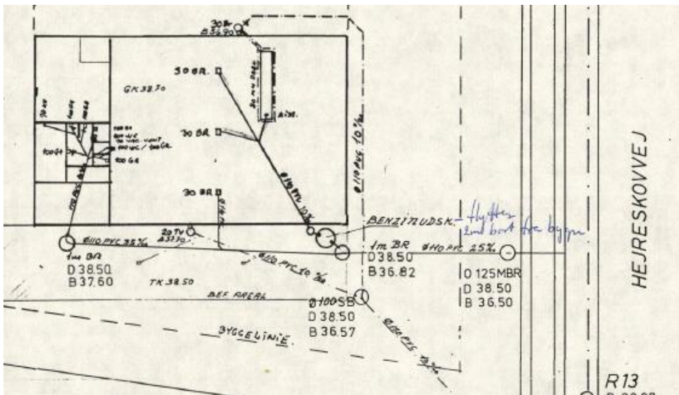
Placering olieudskiller
