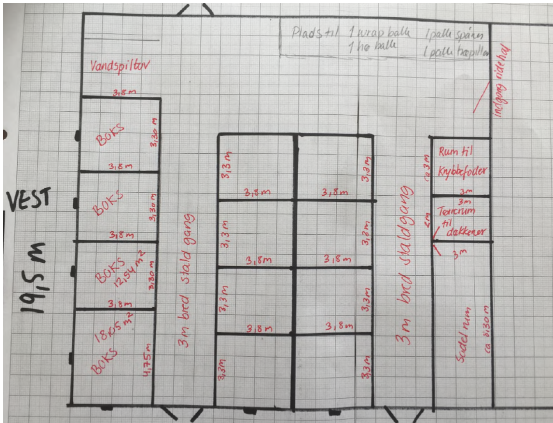
Figur 1: Skitsetegning af hestestald
