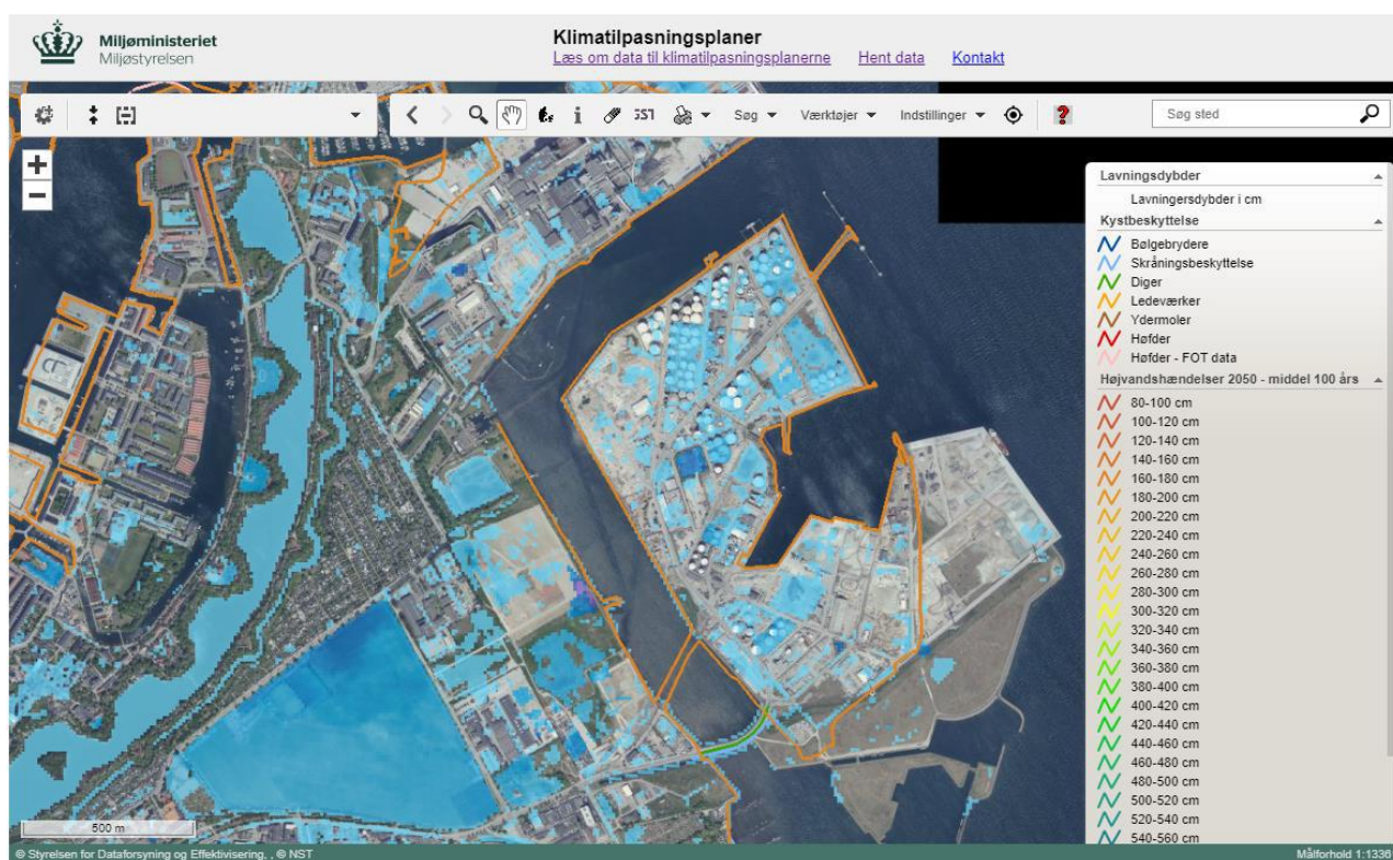
Figur 11 Oversvømmelser ved en 100 årshændelse
