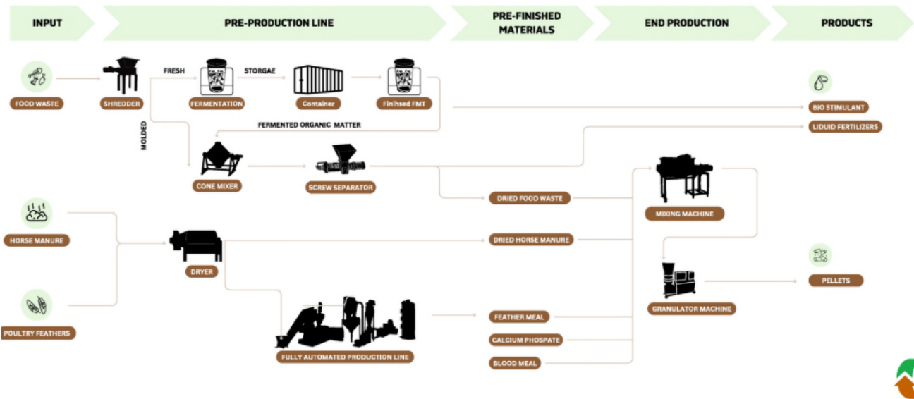
Figur 10 viser flowdiagram for produktionen
