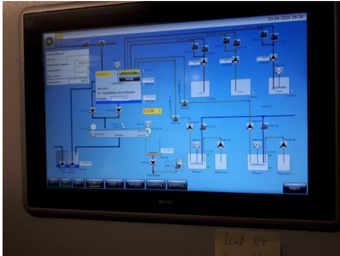
SRO – Styring, Regulering, Overvågning af behandlingsanlægget.
