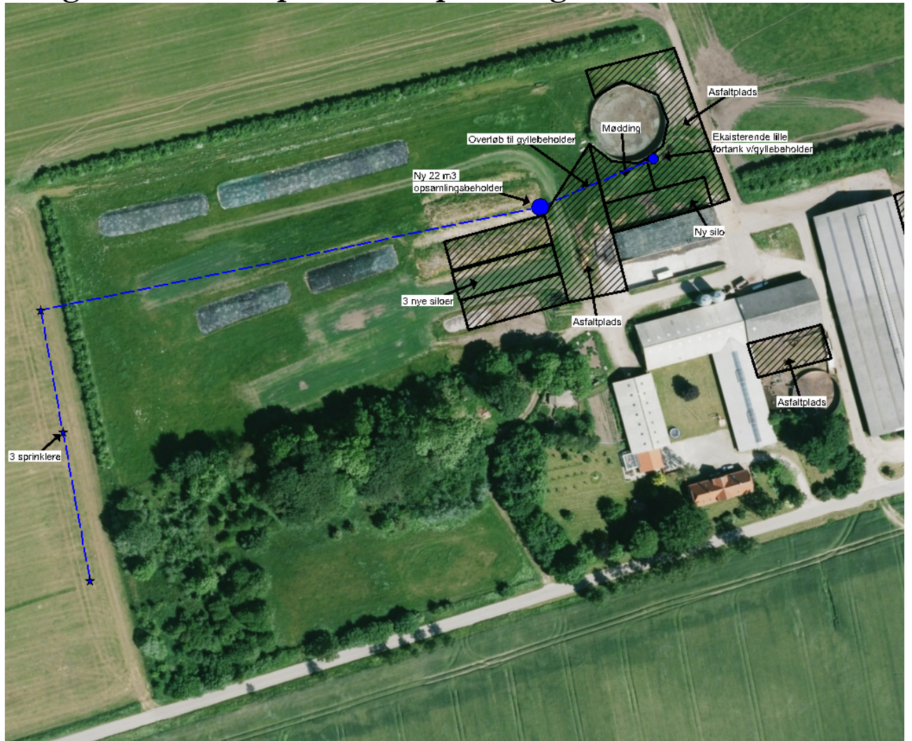
Figur 1. Houtvedvej 5 og det ønskede sprinkleranlæg. Sprinklerne er vist med stjerner til venstre i billedet. Rørforbindelsen er vist med stiptet blå og opsamlingsstanken med en blå cirkel. Ved gyllebeholderen er den lille fortank vist med en blå cirkel. Resten af situationsplanen er kopieret fra den nylige miljøgodkendelse.
