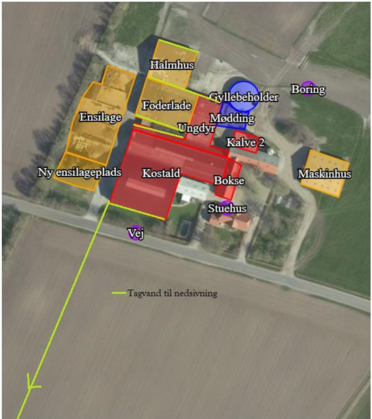
Afløbsplan
