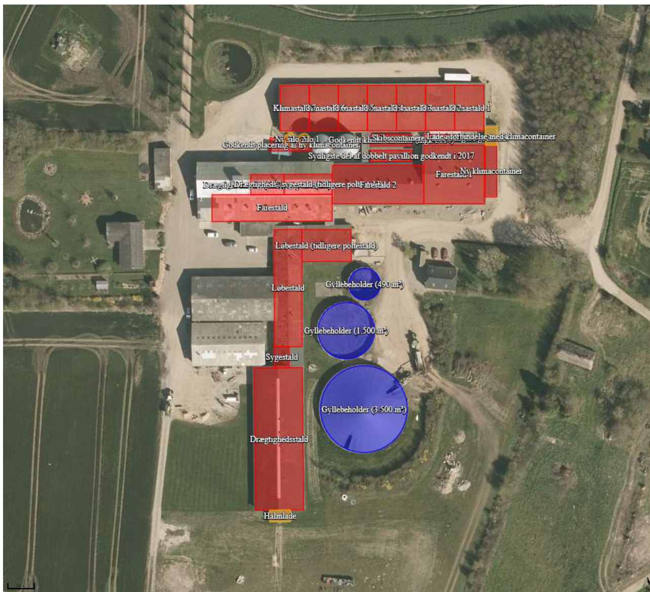
Figur 1: Husdyrbrugets stalde, opbevaringsanlæg mv.
