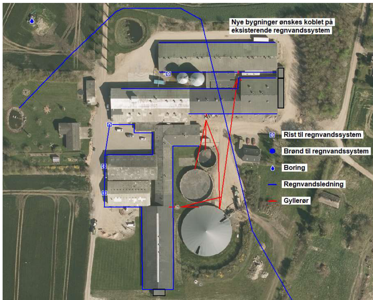
Figur 14: Ledningsplan
