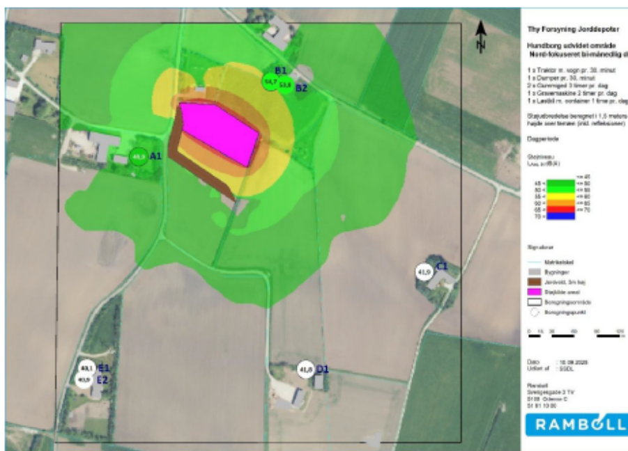
Figur 7-6. Bi-månedlig drift (tømning af område) på den nordlige halvdel af det udvidede projektområde. Støj beregnet i udvalgte beregningspunkter og som støjdbredelse i hele området.
