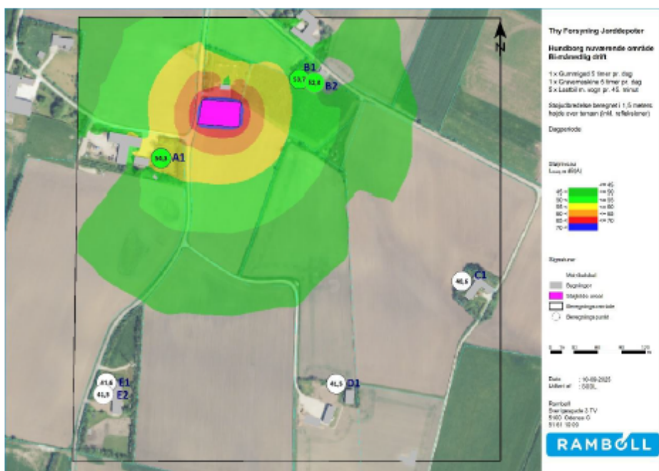
Figur 7-2. Bi-månedlig drift (tømning af område) på det nuværende benyttede område uden jordvold. Støj beregnet i udvalgte beregningspunkter og som støjdbredelse i hele området.
