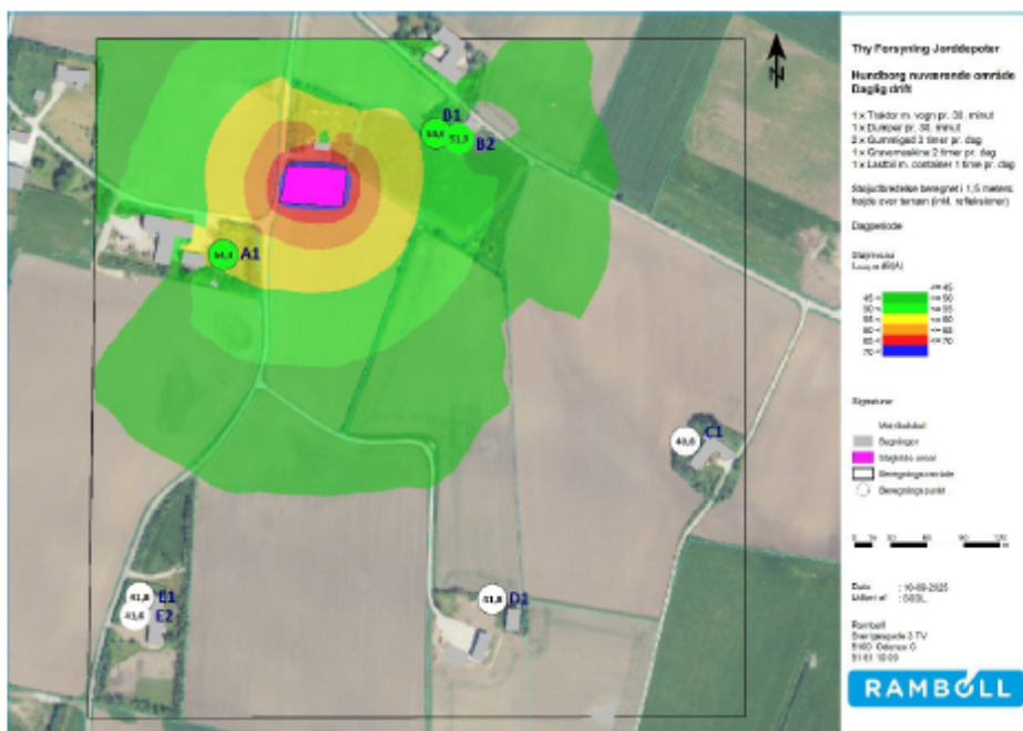
Figur 7-1. Daglig drift (tømning af område) på det nuværende benyttede område uden jordvold. Støj beregnet i udvalgte beregningspunkter og som støjdbredelse i hele området.
