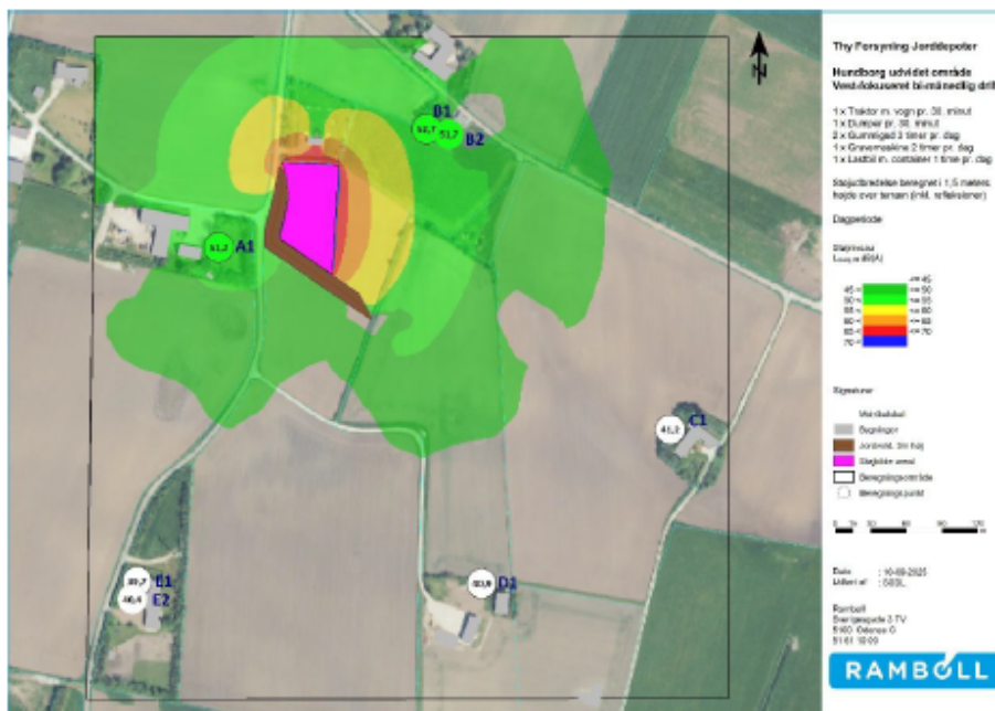
Figur 7-5. Bi-månedlig drift (tømning af område) på den vestlige halvdel af det udvidede projektområde. Støj beregnet i udvalgte beregningspunkter og som støjdbredelse i hele området.
