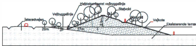
Snit, hvor golfbanen er i lavere niveau, end vejen. Støjvolden er trukket tilbage fra vejbyggefløjen i Hft. reglerne om "tilæg for højdeforskel" jvf. lov om asfalterede veje §40, stk. 5.
