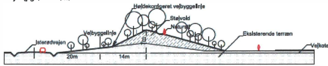
Snit, hvor golfbanen er i højere niveau, end vejen. Støjvolden er trukket tilbage fra vejbyggefløjen i Hft. reglerne om "tilæg for højdeforskel" jvf. lov om asfalterede veje §40, stk. 5.
