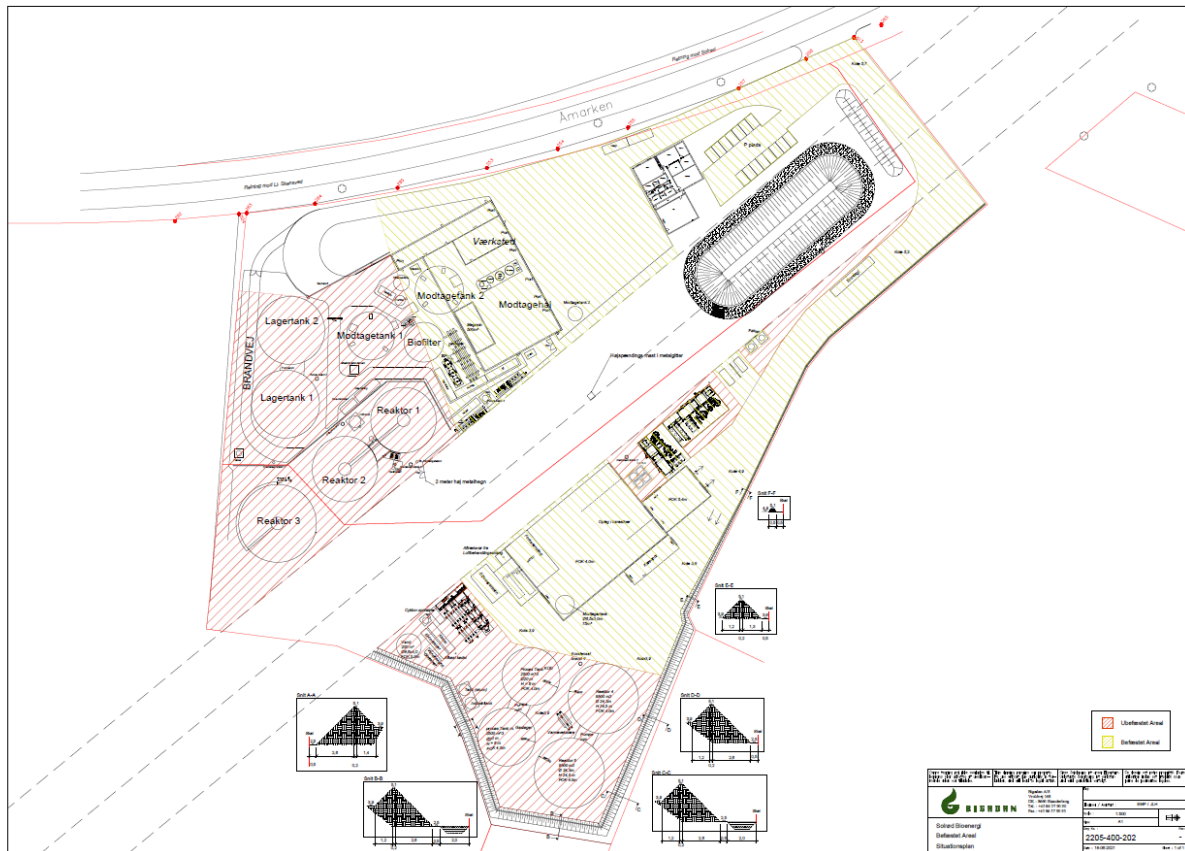
Figur 1: Anlægsskitse med markering af afstrømningsoplande på SOLRØD BIOGAS A/S og Solrød Bioenergi markeret med henholdsvis rød og gul. Arealet markeret med gult er befæstet. Arealet markeret med rødt er ubefæstet.
